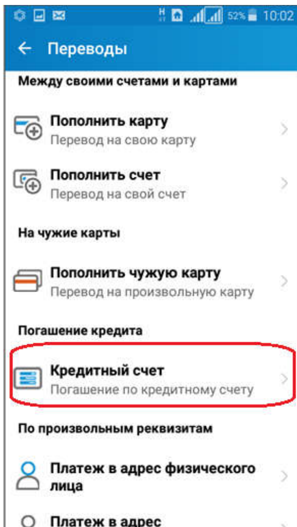
Выбор перевода
