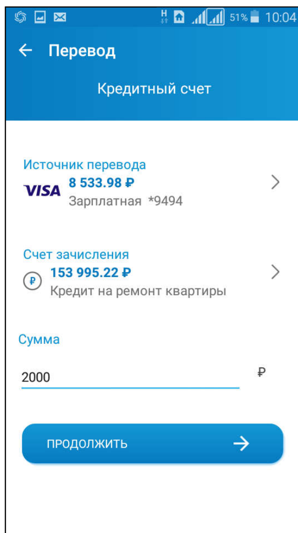
Создание перевода
